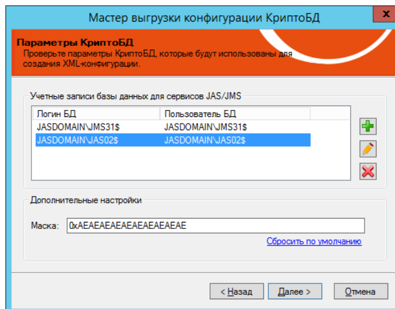
Рис. 280 – Окно задания учетных записей для работы СКЗИ «Крипто БД» с БД JMS
