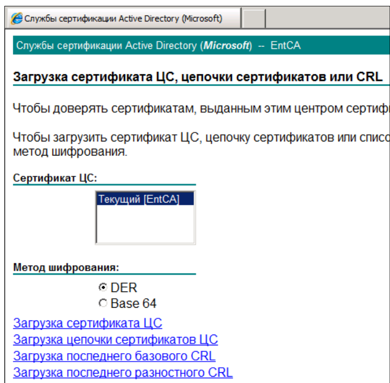
Рис. 158 – Страница загрузки сертификата центра сертификации Microsoft
