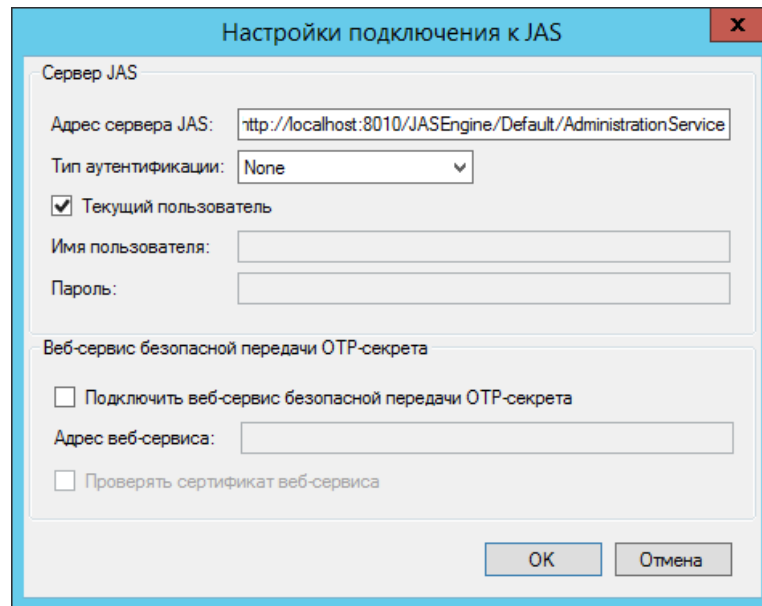
Рис. 229 – Окно настроек подключения к JAS
