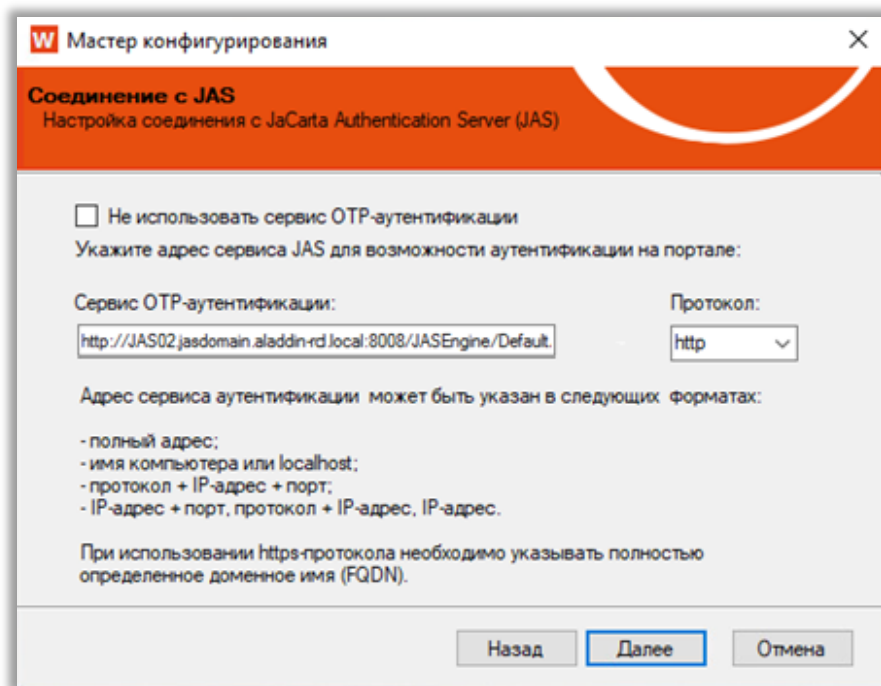
Рис. 242 – Окно настройки подключения к серверу JAS
