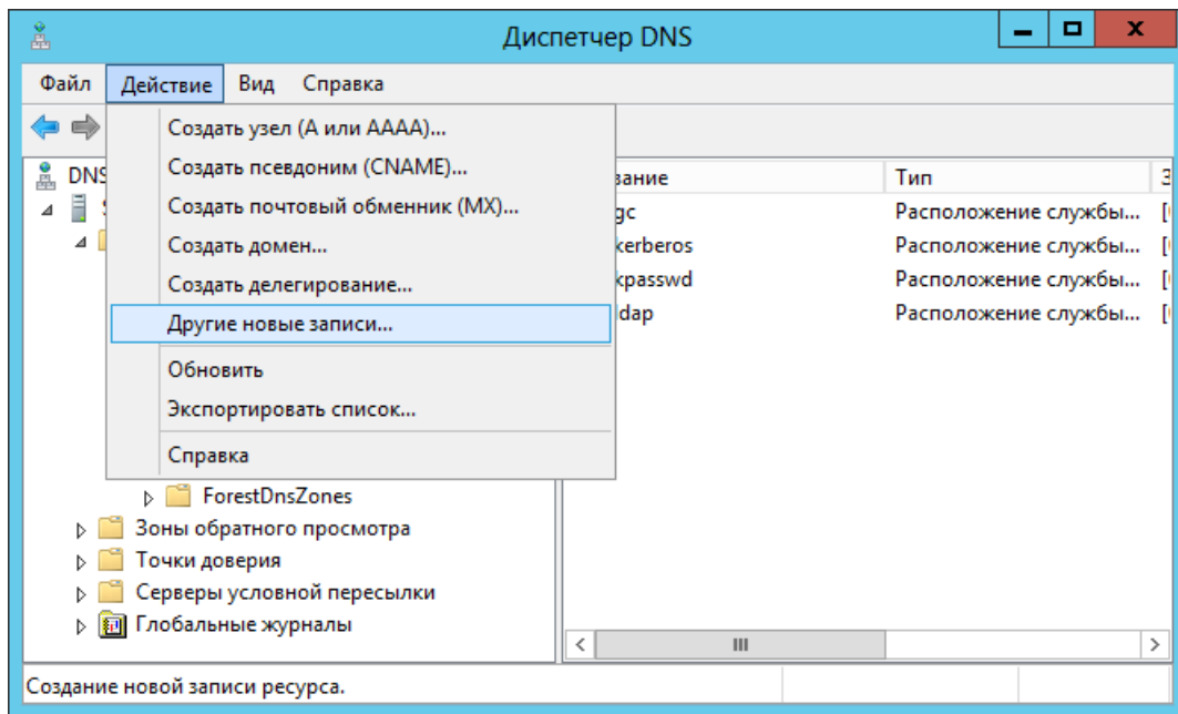
Рис. 132 – Создание новой записи
