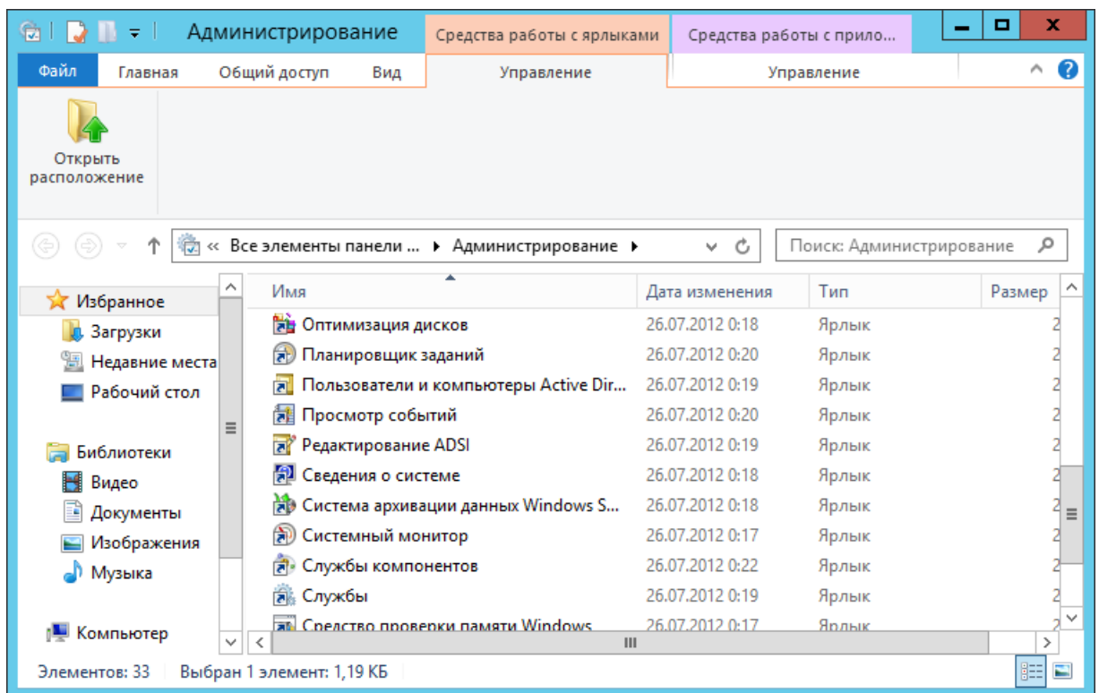
Рис. 70 – Возможности администрирования
