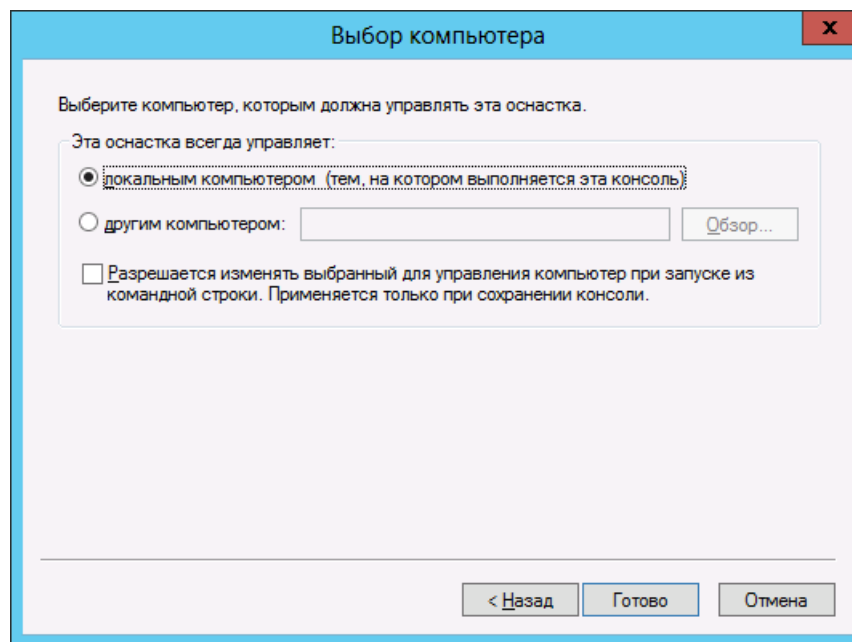
Рис. 31 – Выбор компьютера
