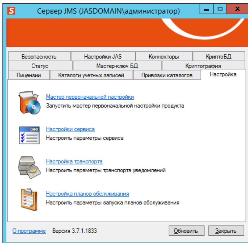
Рис. 77 – Вкладка Настройка
