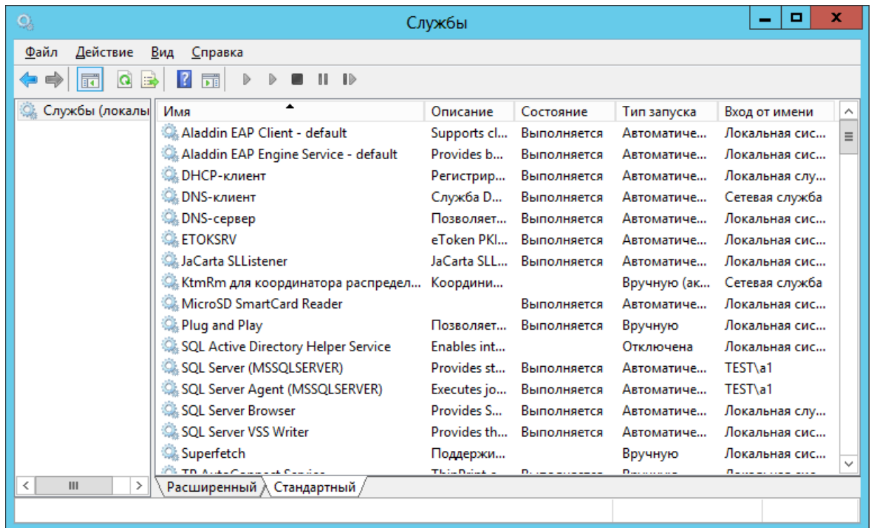
Рис. 74 – Список служб
