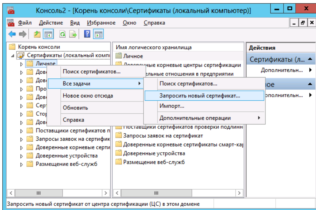
Рис. 33 – Запрос сертификата
