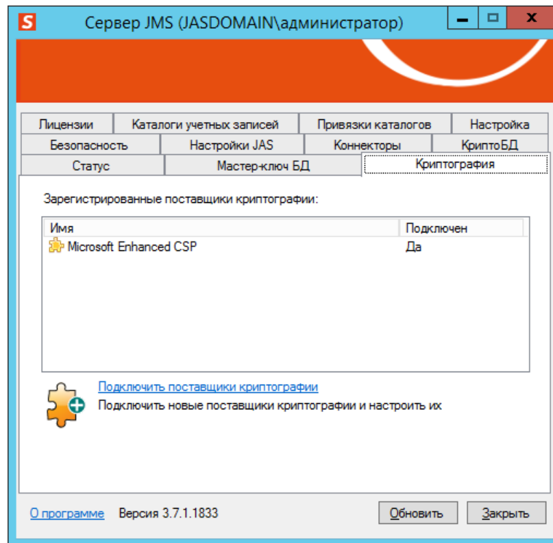
Рис. 195 – Вкладка Криптография
