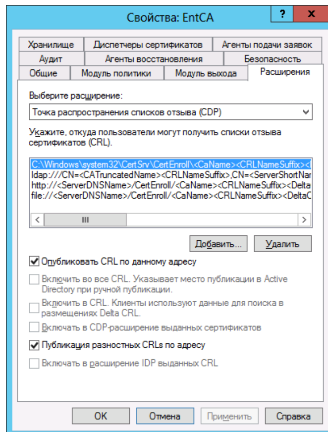
Рис. 2 – Вкладка Расширения
