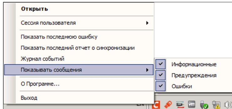
Рис. 164 – Включение/отключение уведомлений
