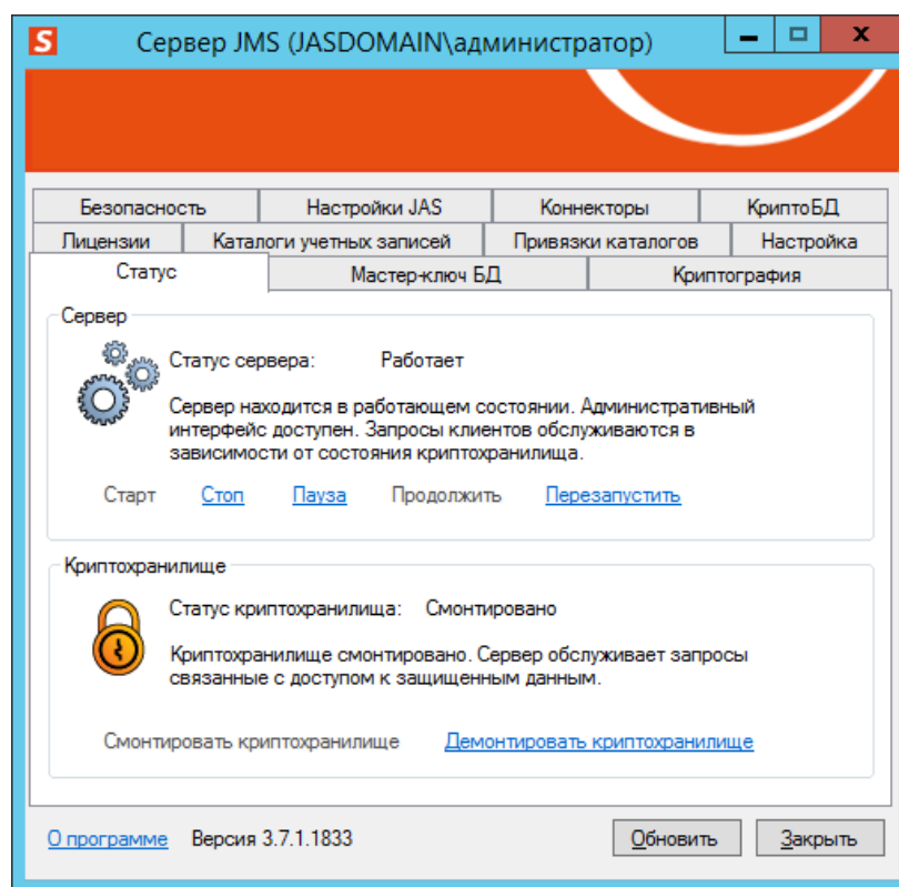
Рис. 166 – Вкладка Статус
