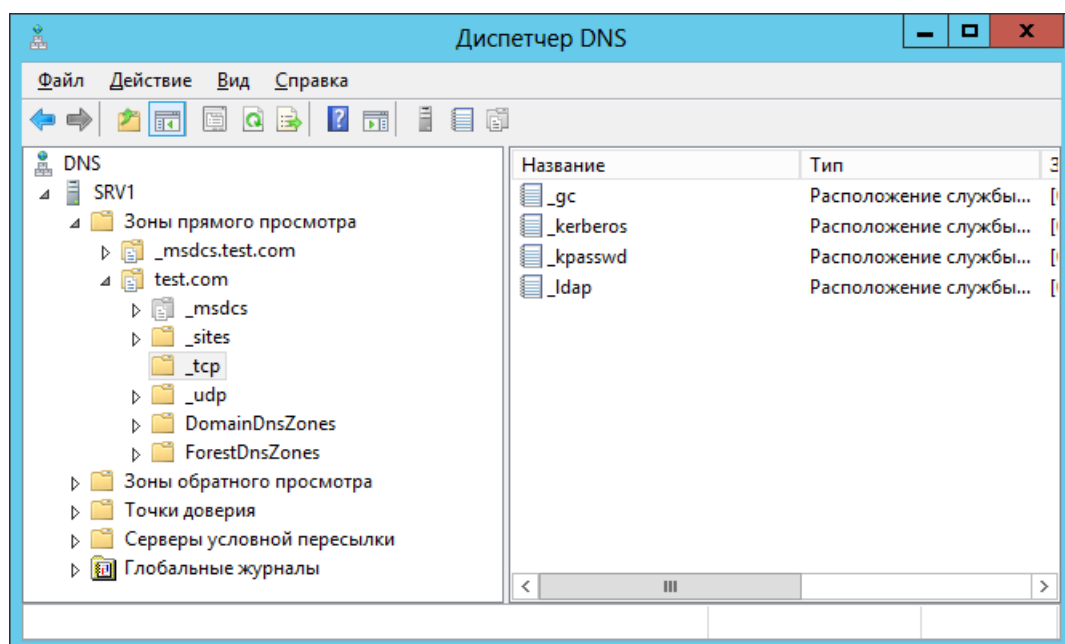
Рис. 131 – Выбор протокола
