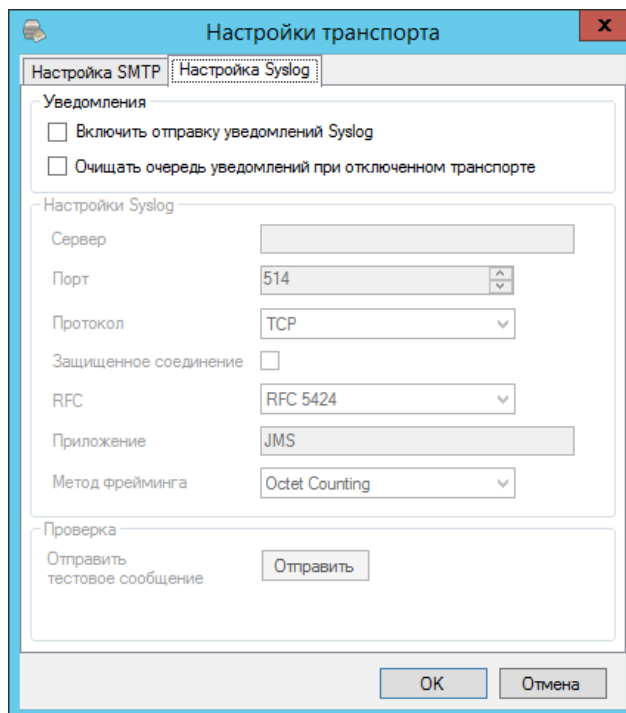
Рис. 220 – Настройка Syslog
