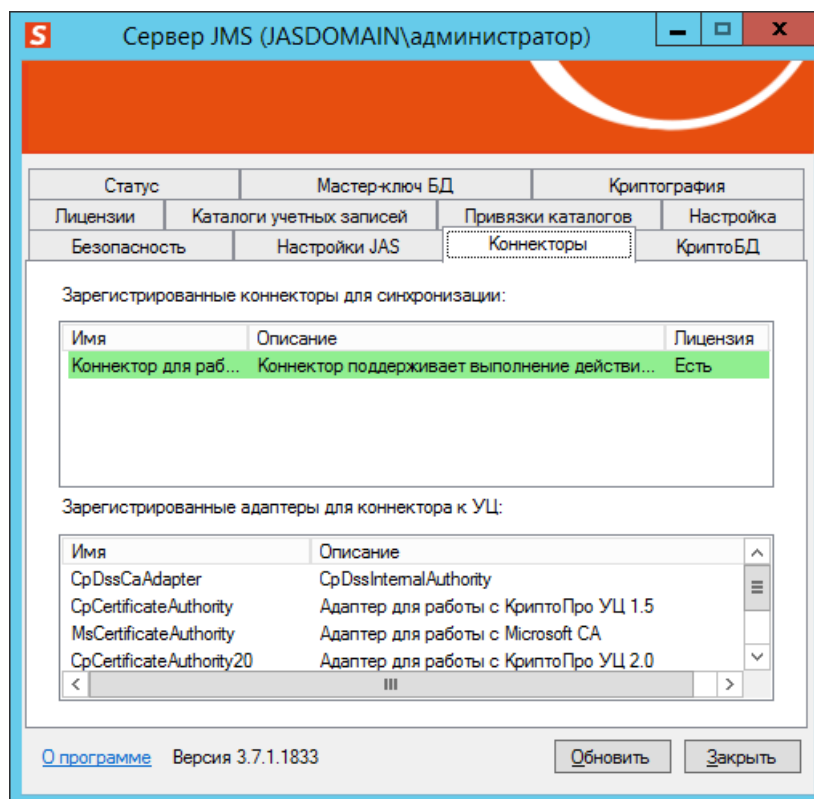
Рис. 227 – Вкладка Коннекторы
